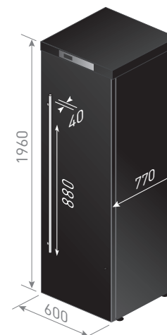
Dimensions en mm
